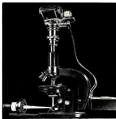
Micro-tussenstuk en lichtintensiteitsmete
