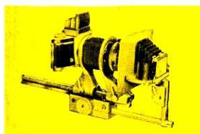
Dia-copieerinrichting aan het balgapparaat met instelslede
