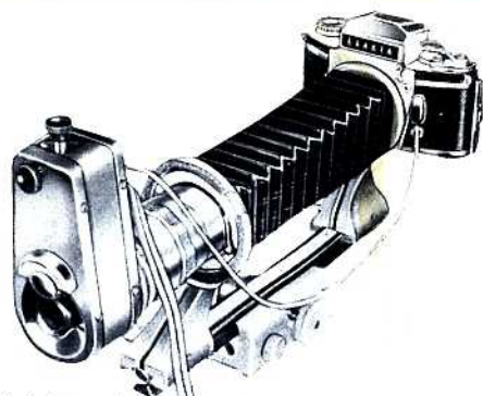
Kolpofot met elektronische ringlamp RB 1
