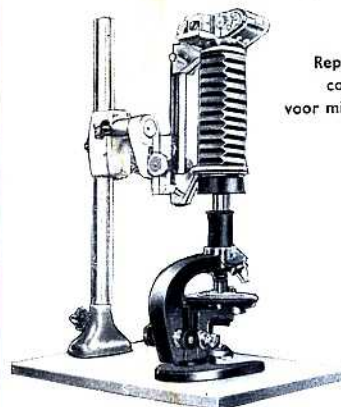
Micro-tussenstuk en lichtintensiteitsmeter
